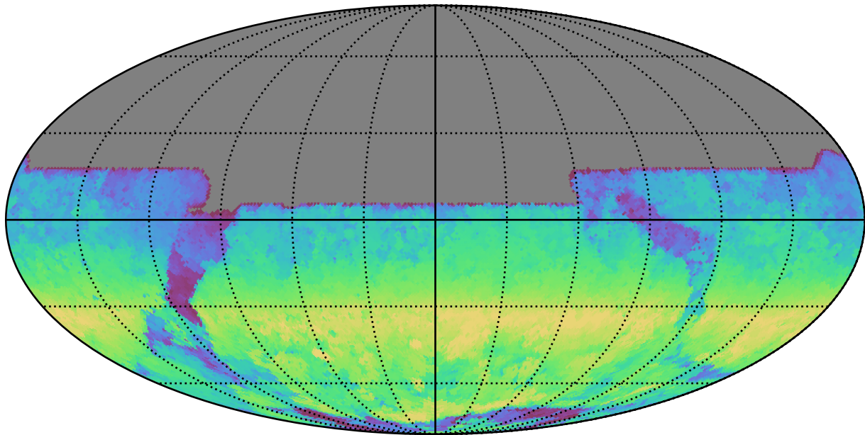
no_high_blob_v3.3_10yrs All sky y band: AngleRange rotSkyPos
