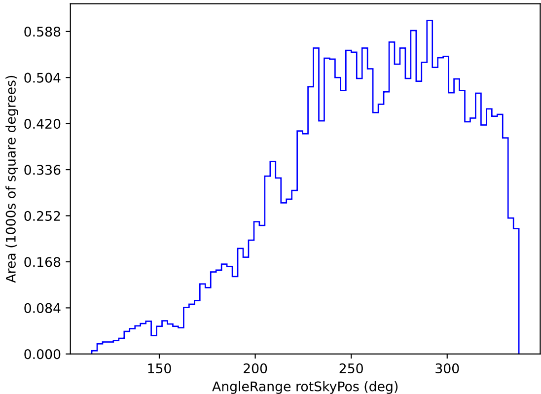
no_high_blob_v3.3_10yrs All sky y band: AngleRange rotSkyPos
