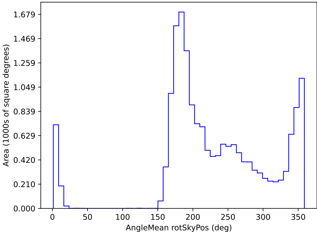
no_high_blob_v3.3_10yrs WFD y band: AngleMean rotSkyPos
