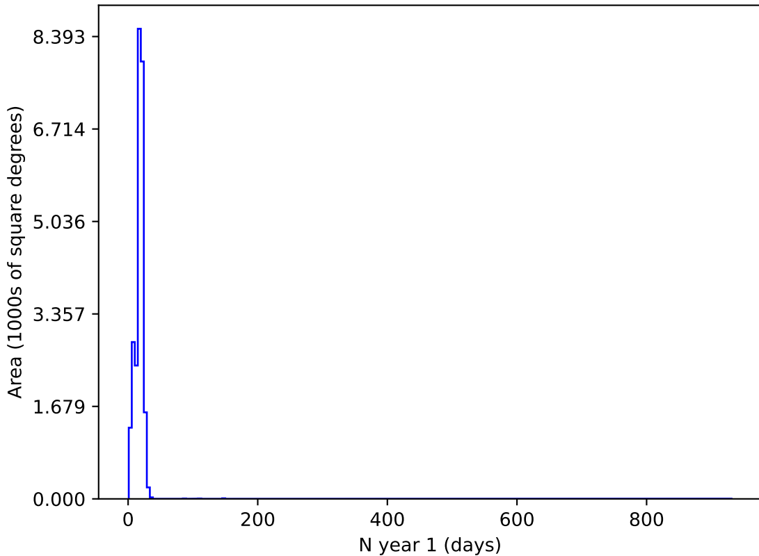
no_high_blob_v3.3_10yrs y and night < 365: N year 1
