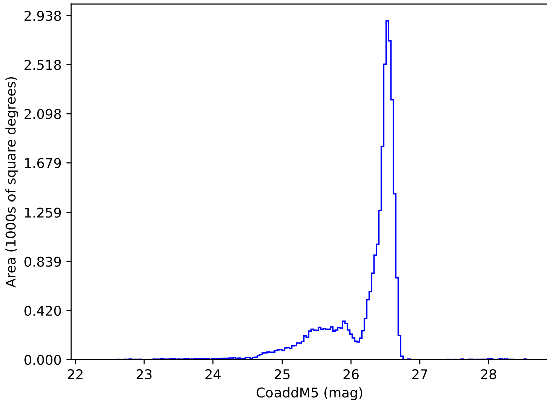
no_high_blob_v3.3_10yrs i: CoaddM5
