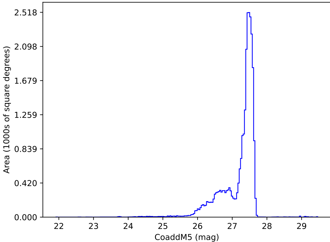
no_high_blob_v3.3_10yrs : CoaddM5
