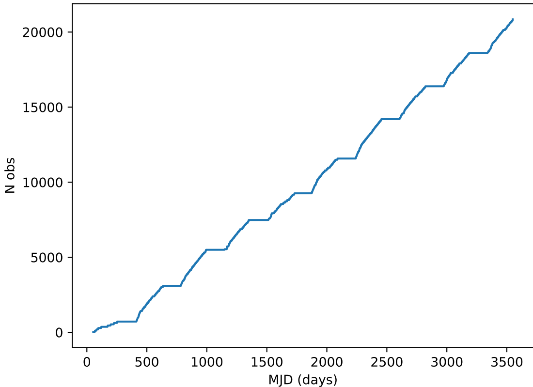
no_high_blob_v3.3_10yrs all bands: DD:ELAISS1 Cumulative NVisits
