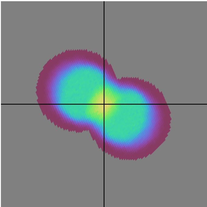
no_high_blob_v3.3_10yrs z band: DD:EDFS NVisits
