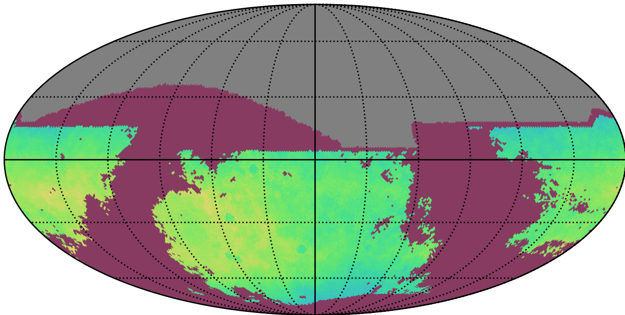
mw_roll_bulge_v3.3_10yrs i: NgalScale
