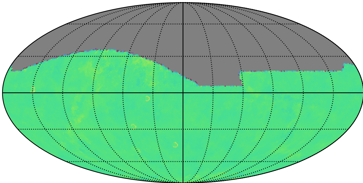
mw_roll_bulge_v3.3_10yrs z: Kuiper rotTelPos
