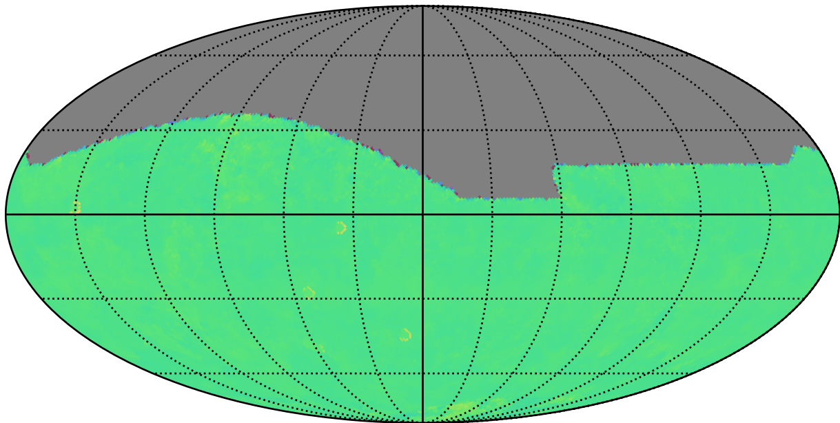
mw_roll_bulge_v3.3_10yrs i: Kuiper rotTelPos
