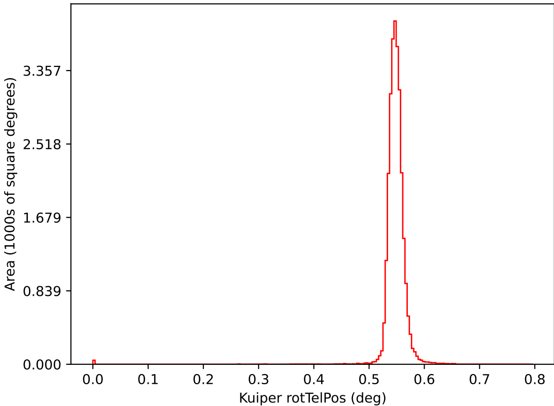
mw_roll_bulge_v3.3_10yrs i: Kuiper rotTelPos
