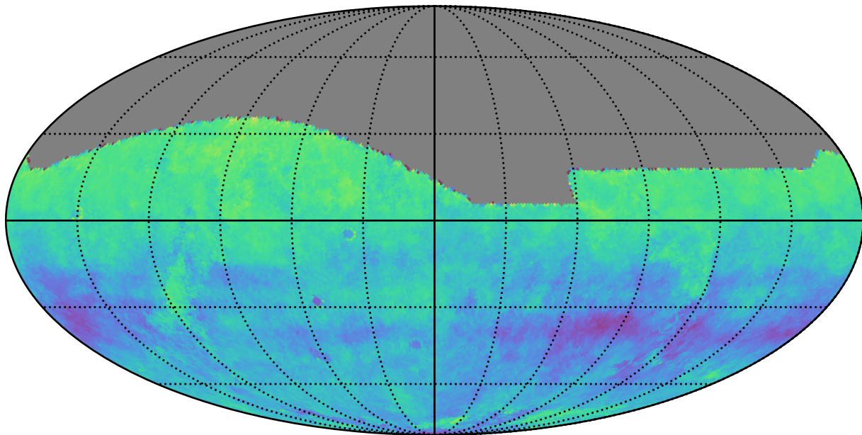
mw_roll_bulge_v3.3_10yrs i: Kuiper rotSkyPos
