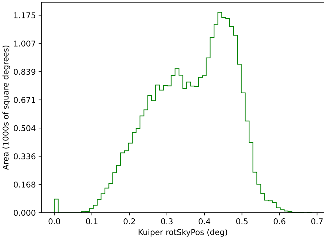
mw_roll_bulge_v3.3_10yrs g: Kuiper rotSkyPos
