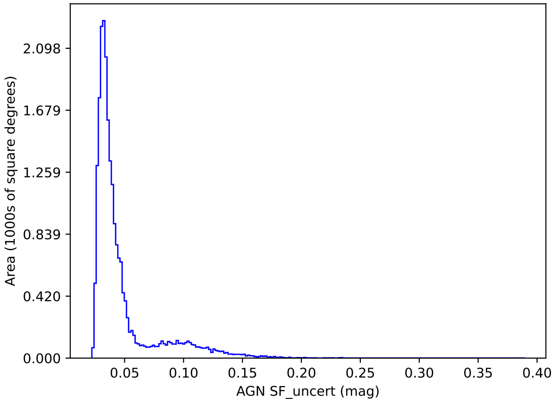
mw_roll_bulge_v3.3_10yrs y band: AGN SF_uncert
