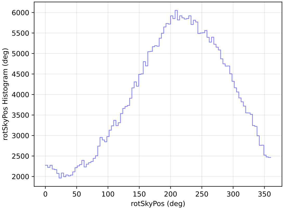
mw_roll_bulge_v3.3_10yrs WFD y band: rotSkyPos Histogram
