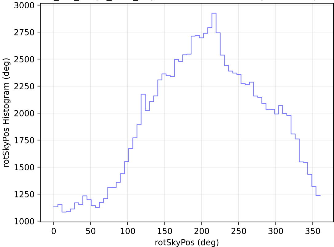
mw_roll_bulge_v3.3_10yrs WFD u band: rotSkyPos Histogram
