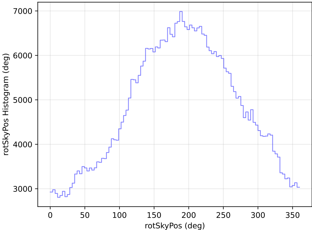
mw_roll_bulge_v3.3_10yrs WFD r band: rotSkyPos Histogram
