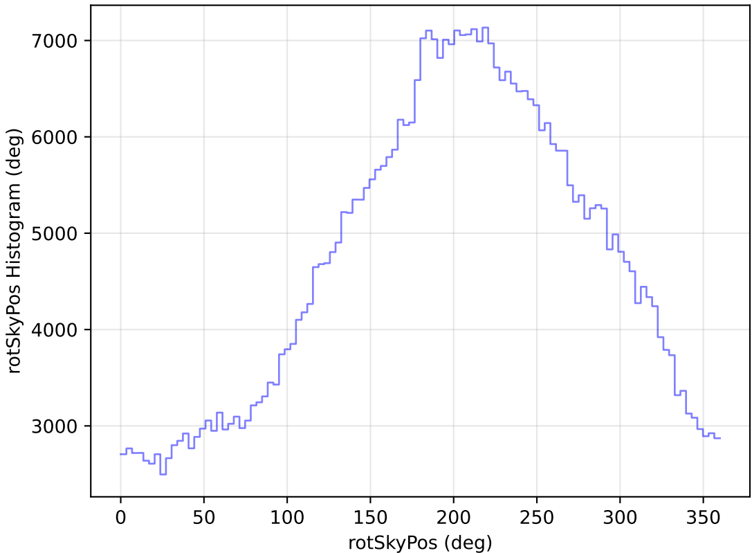
mw_roll_bulge_v3.3_10yrs WFD i band: rotSkyPos Histogram
