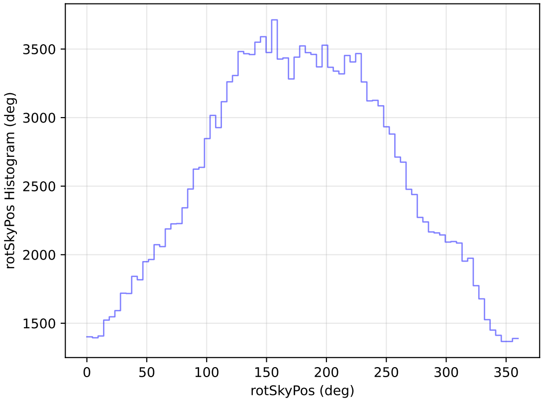
mw_roll_bulge_v3.3_10yrs WFD g band: rotSkyPos Histogram
