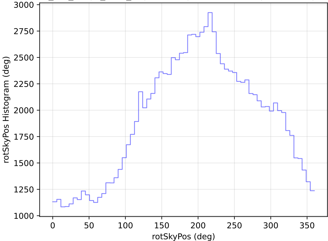
mw_roll_bulge_v3.3_10yrs All sky u band: rotSkyPos Histogram
