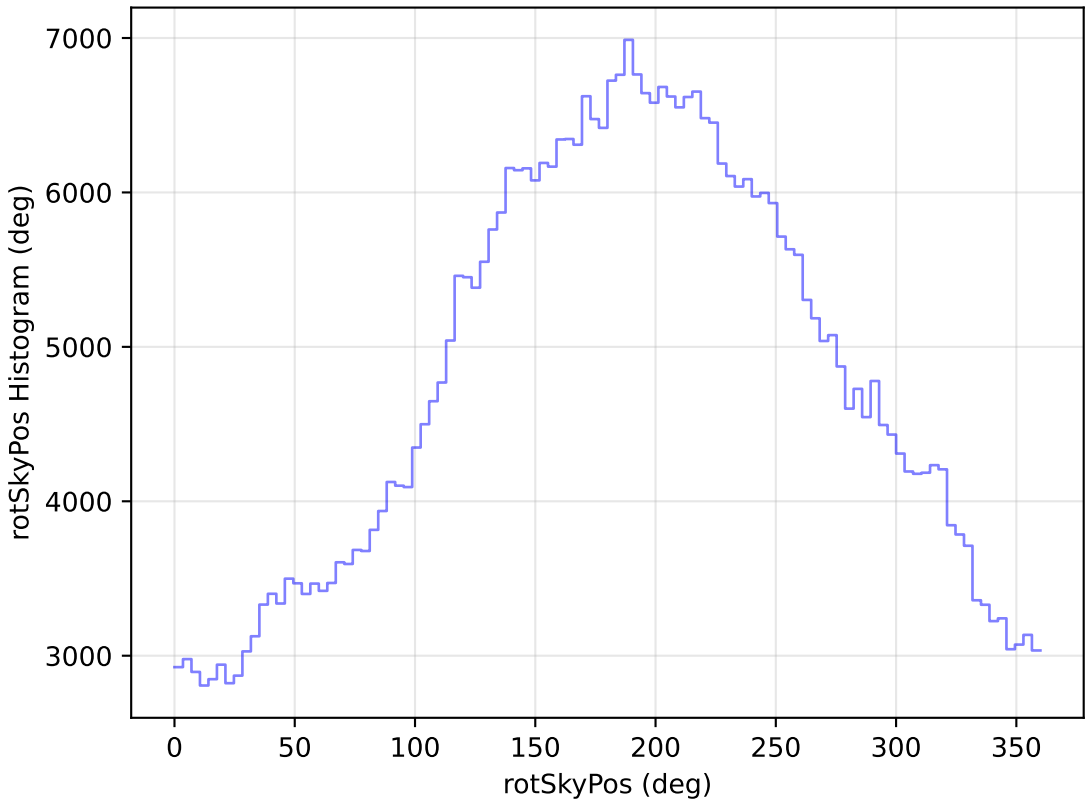
mw_roll_bulge_v3.3_10yrs All sky r band: rotSkyPos Histogram
