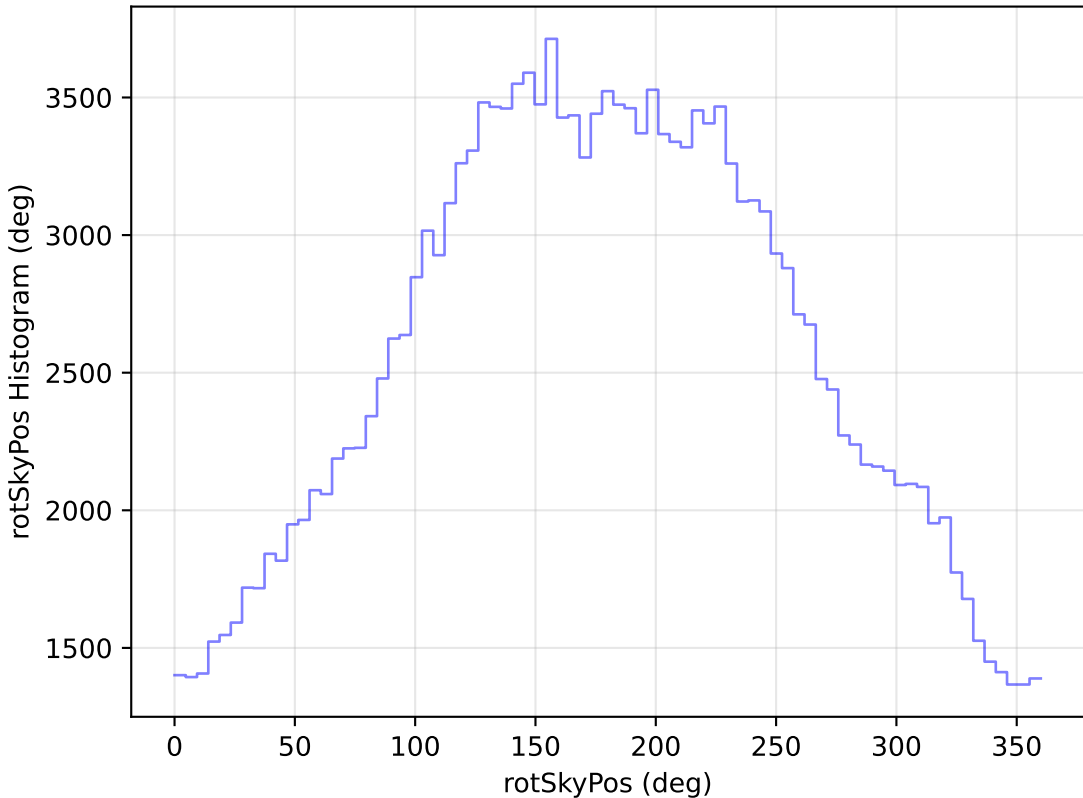
mw_roll_bulge_v3.3_10yrs All sky g band: rotSkyPos Histogram
