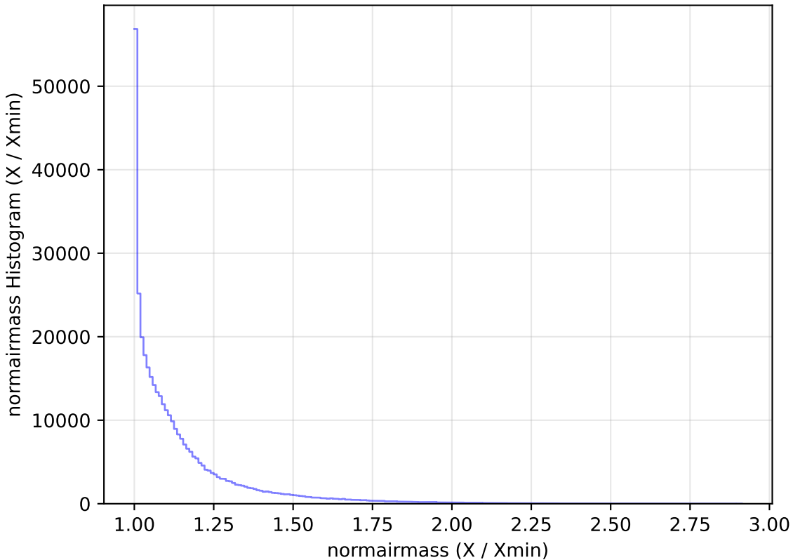
mw_roll_bulge_v3.3_10yrs All sky y band: normairmass Histogram
