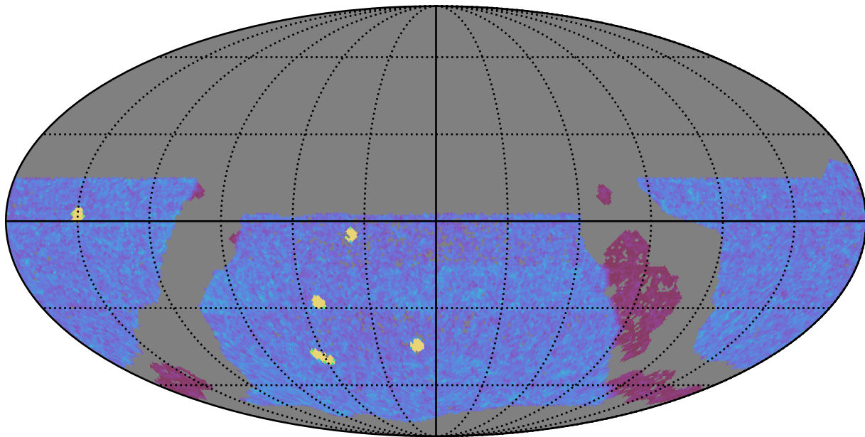
mw_roll_bulge_v3.3_10yrs WFD y band: NVisits
