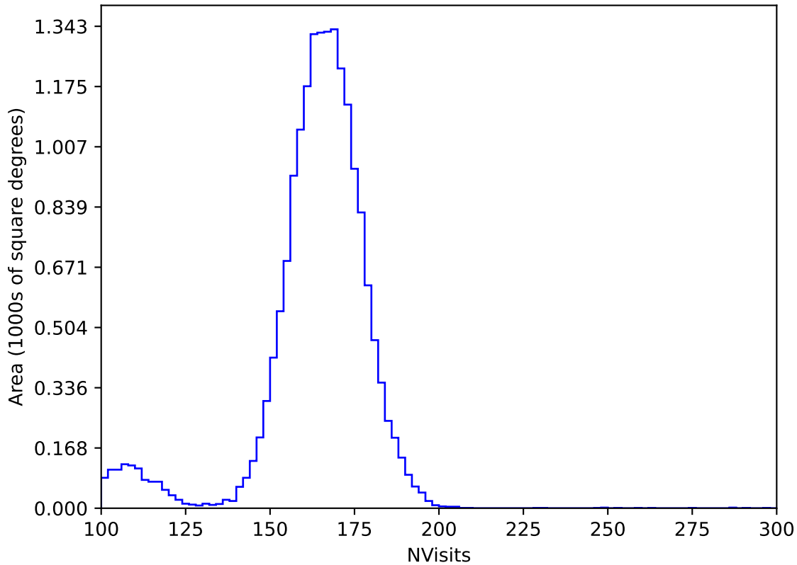
mw_roll_bulge_v3.3_10yrs WFD y band: NVisits
