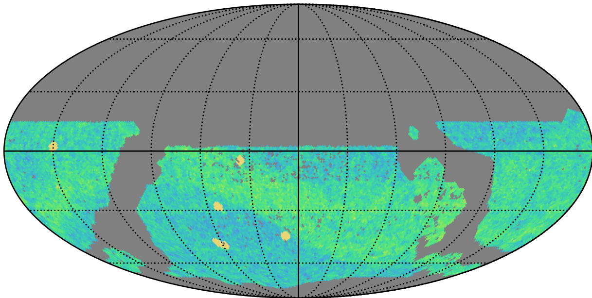
mw_roll_bulge_v3.3_10yrs WFD i band: NVisits
