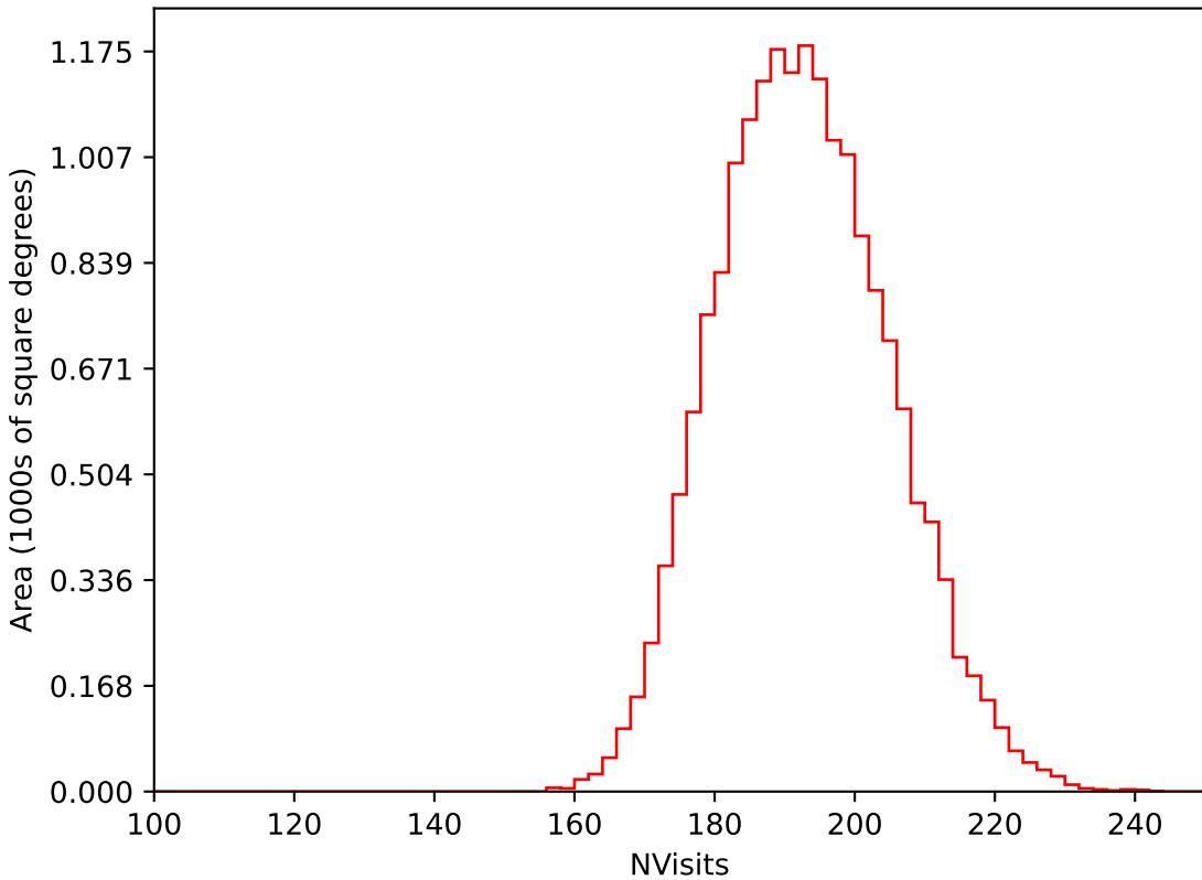
mw_roll_bulge_v3.3_10yrs WFD i band: NVisits
