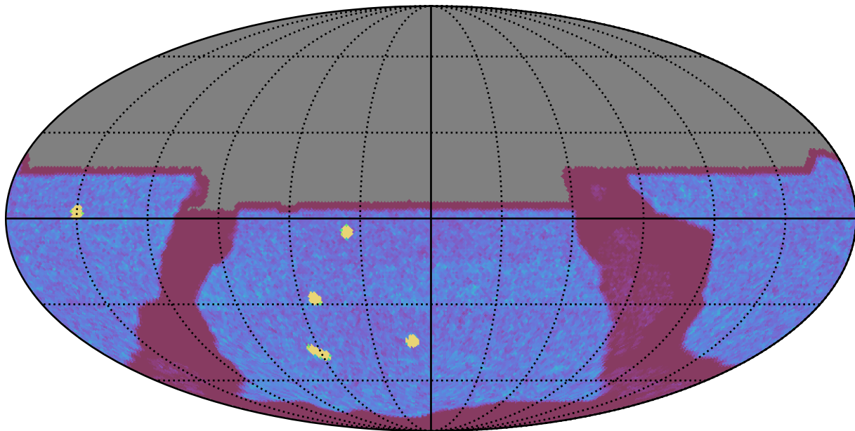
mw_roll_bulge_v3.3_10yrs All sky y band: NVisits
