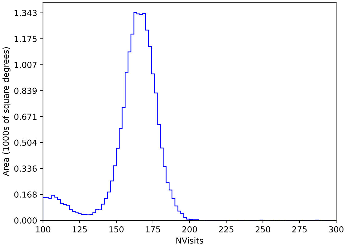
mw_roll_bulge_v3.3_10yrs All sky y band: NVisits
