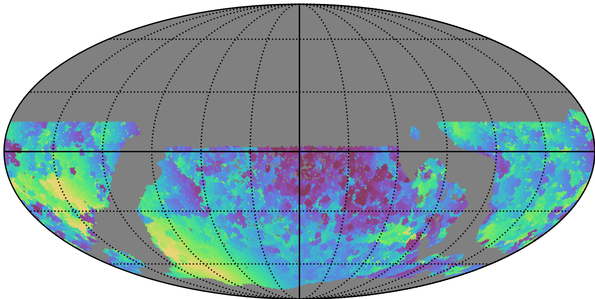
mw_roll_bulge_v3.3_10yrs WFD y band: Min solarElong
