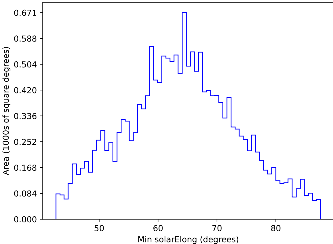
mw_roll_bulge_v3.3_10yrs WFD y band: Min solarElong
