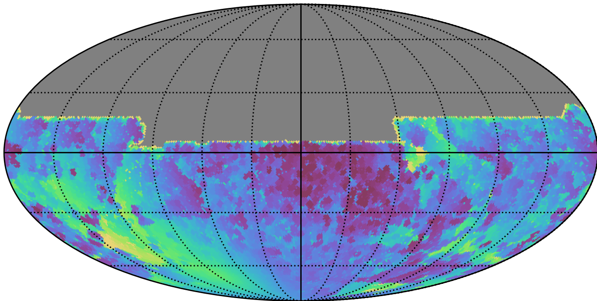
mw_roll_bulge_v3.3_10yrs All sky y band: Min solarElong
