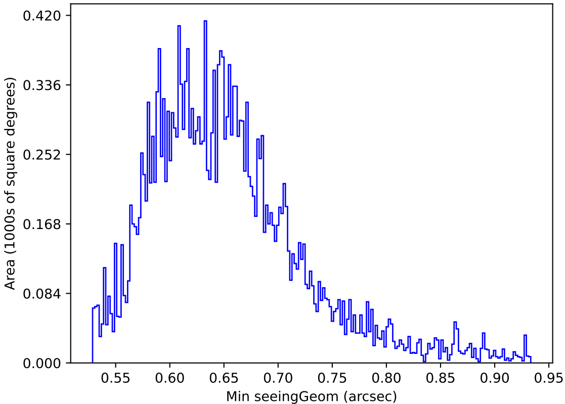
mw_roll_bulge_v3.3_10yrs Yr 1 y band: Min seeingGeom
