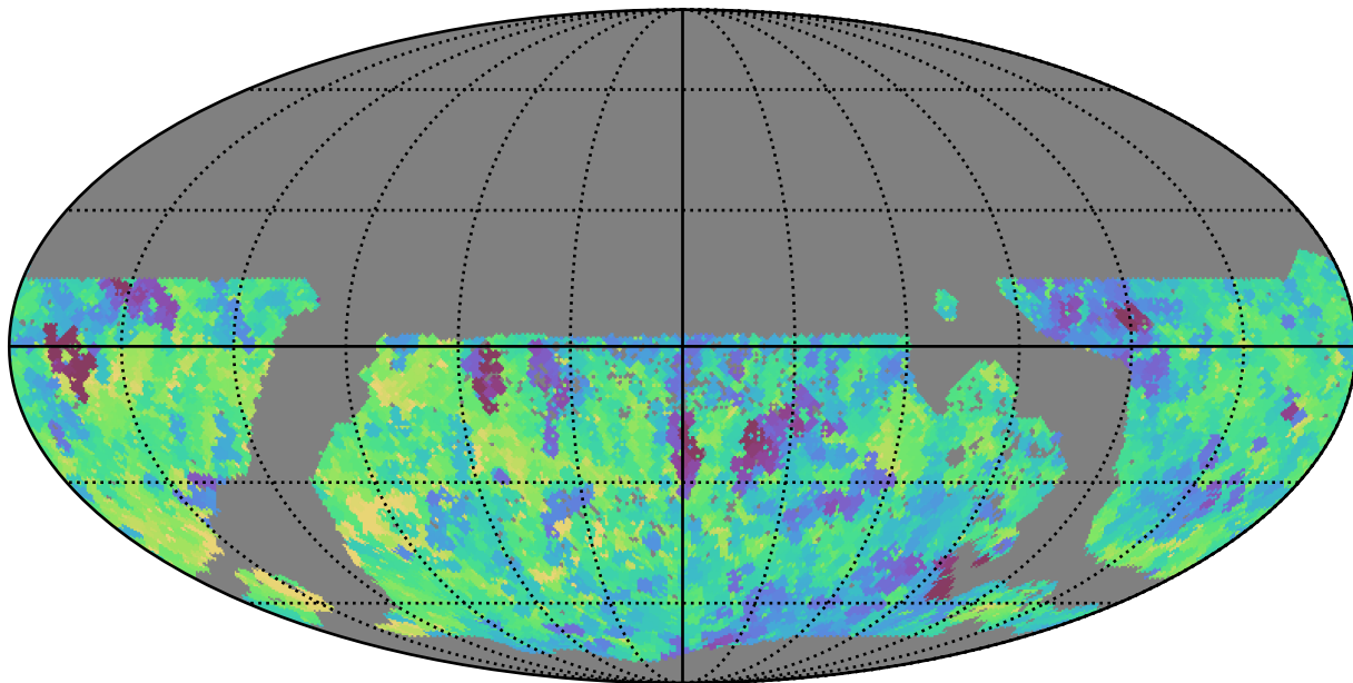
mw_roll_bulge_v3.3_10yrs WFD z band: Min saturation_mag
