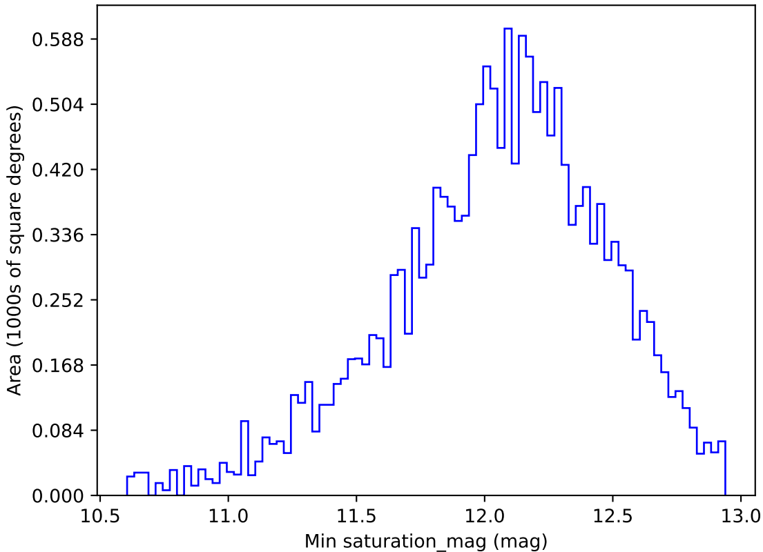
mw_roll_bulge_v3.3_10yrs WFD z band: Min saturation_mag
