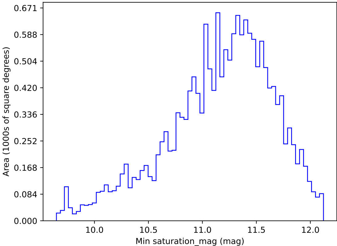
mw_roll_bulge_v3.3_10yrs WFD y band: Min saturation_mag
