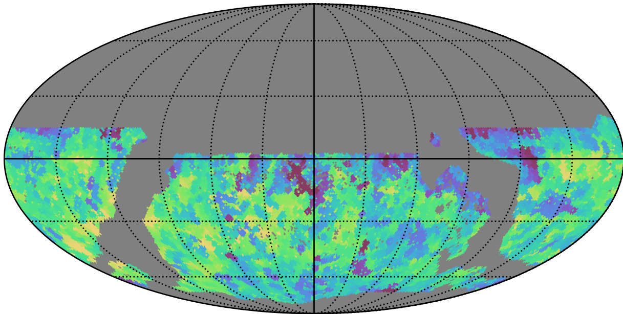
mw_roll_bulge_v3.3_10yrs WFD r band: Min saturation_mag
