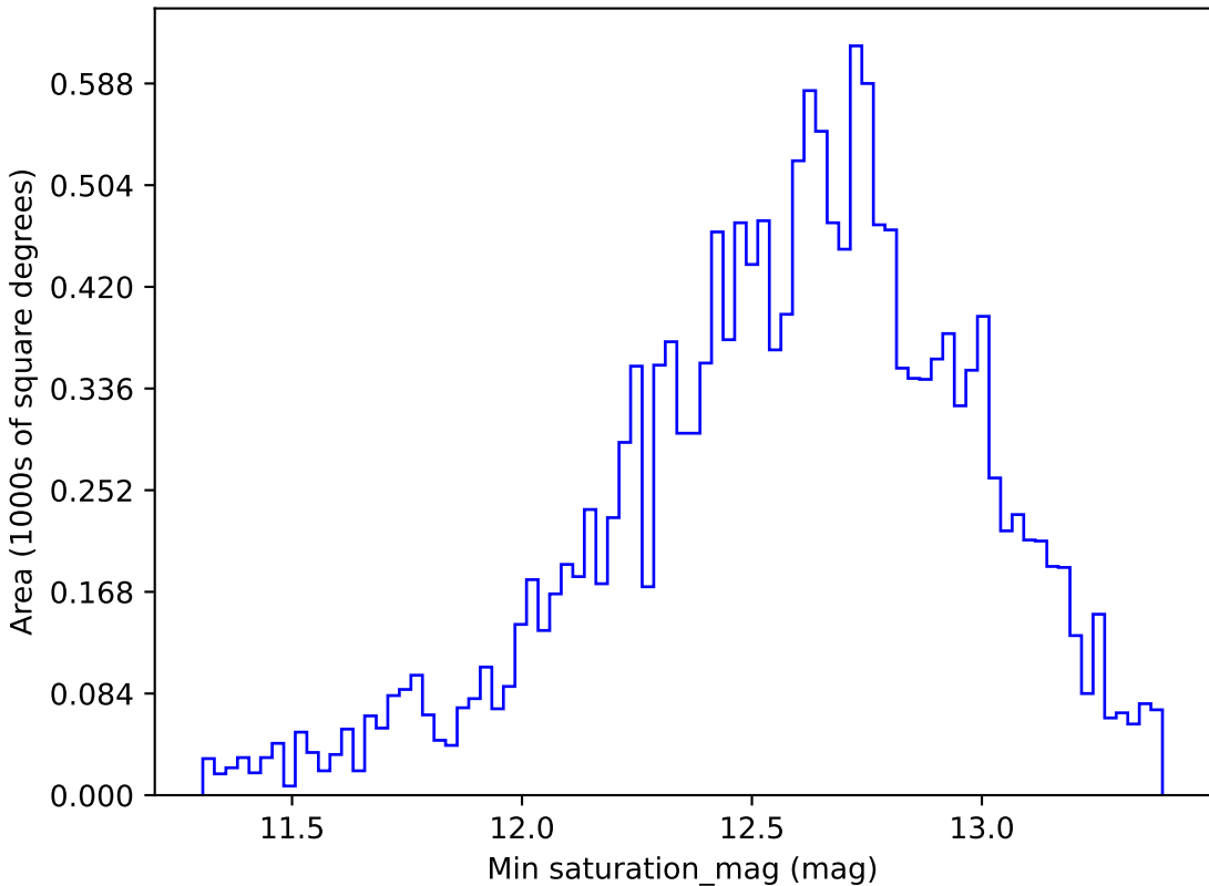
mw_roll_bulge_v3.3_10yrs WFD r band: Min saturation_mag
