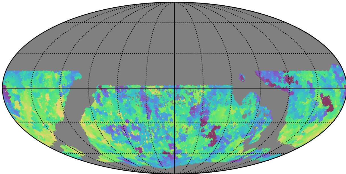
mw_roll_bulge_v3.3_10yrs WFD i band: Min saturation_mag
