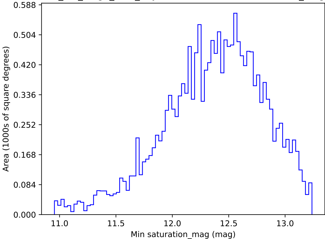
mw_roll_bulge_v3.3_10yrs WFD i band: Min saturation_mag
