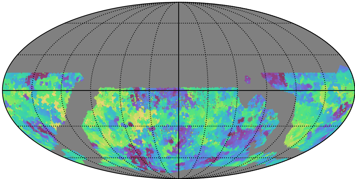
mw_roll_bulge_v3.3_10yrs WFD g band: Min saturation_mag
