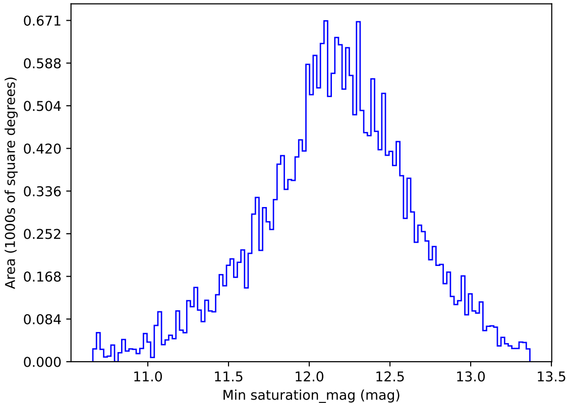
mw_roll_bulge_v3.3_10yrs All sky z band: Min saturation_mag
