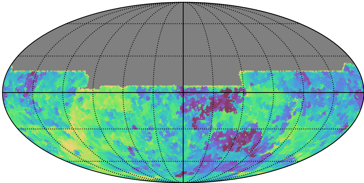
mw_roll_bulge_v3.3_10yrs All sky y band: Min saturation_mag
