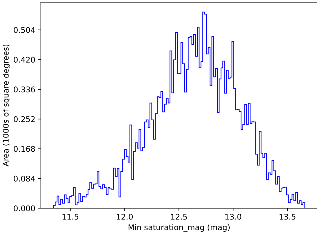
mw_roll_bulge_v3.3_10yrs All sky r band: Min saturation_mag
