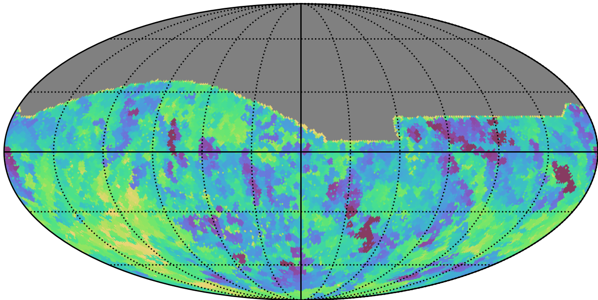
mw_roll_bulge_v3.3_10yrs All sky i band: Min saturation_mag
