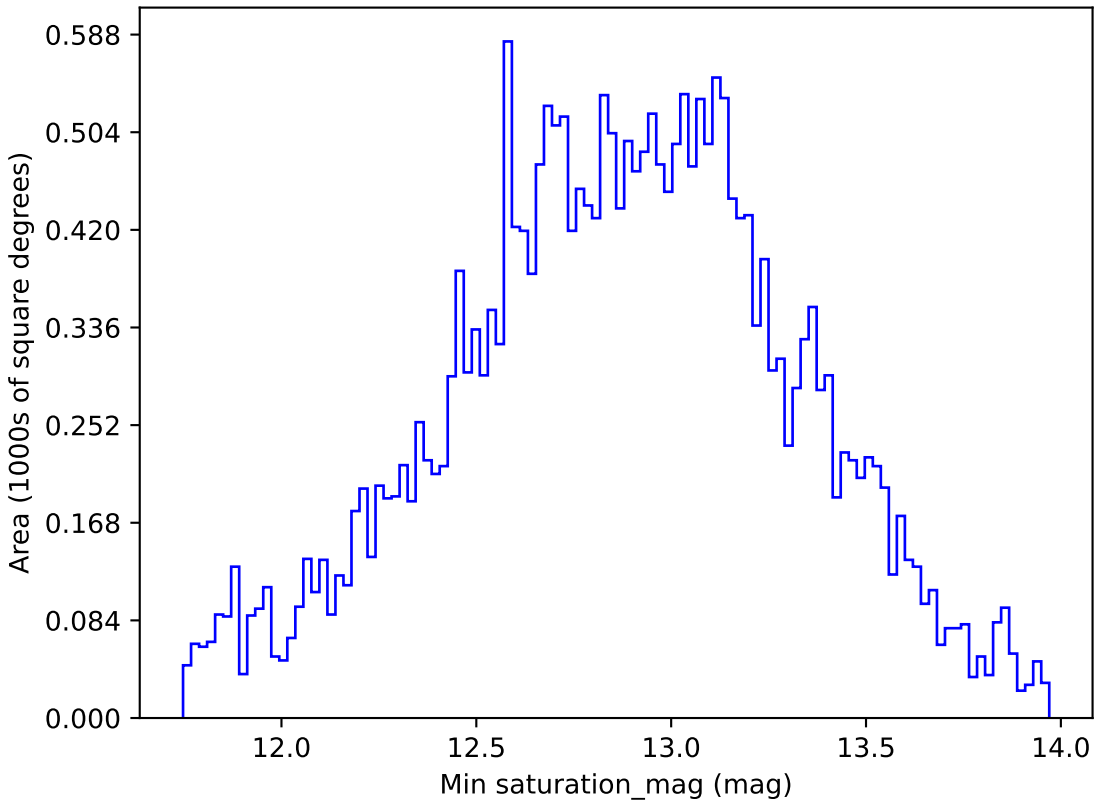
mw_roll_bulge_v3.3_10yrs All sky g band: Min saturation_mag
