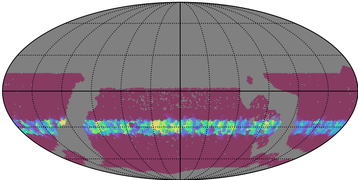
mw_roll_bulge_v3.3_10yrs WFD z band: Min normairmass
