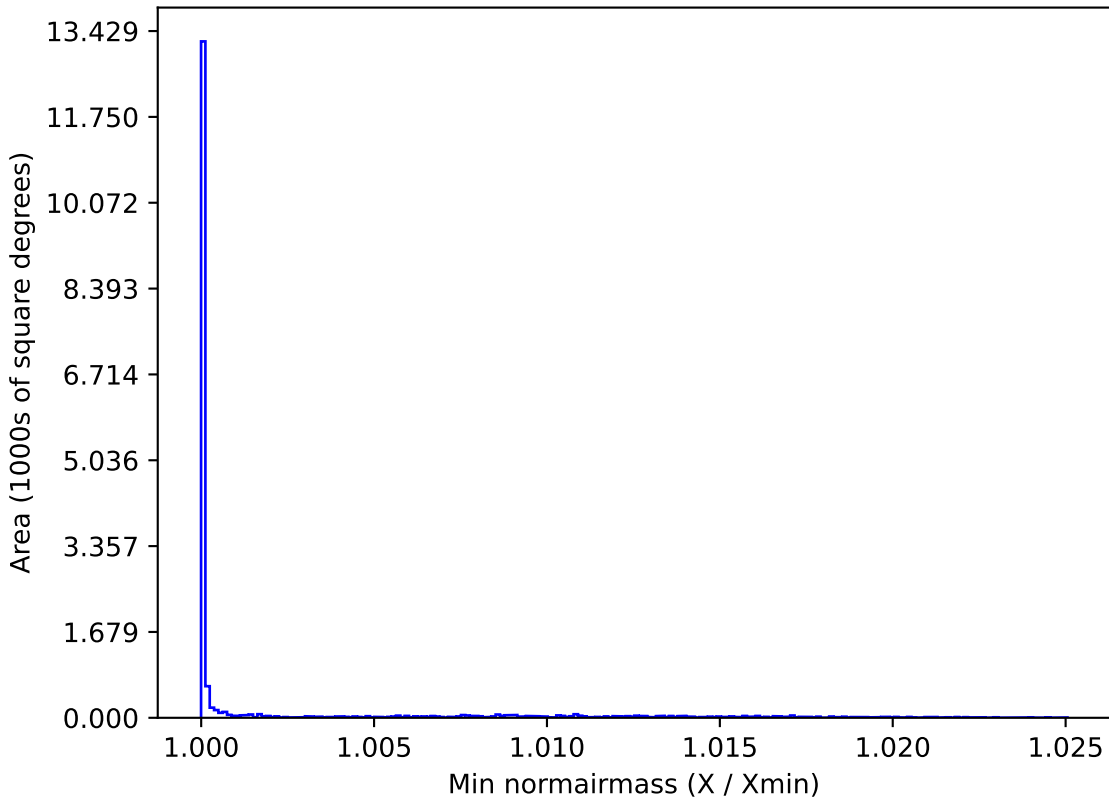
mw_roll_bulge_v3.3_10yrs WFD z band: Min normairmass
