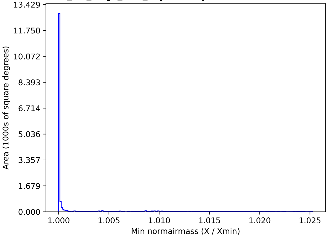
mw_roll_bulge_v3.3_10yrs WFD y band: Min normairmass
